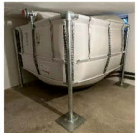
Installationsbsp.: Hargassner Kombianlage Stückgut / Pellets inkl. Sacksilos zur Pelletslagerung
